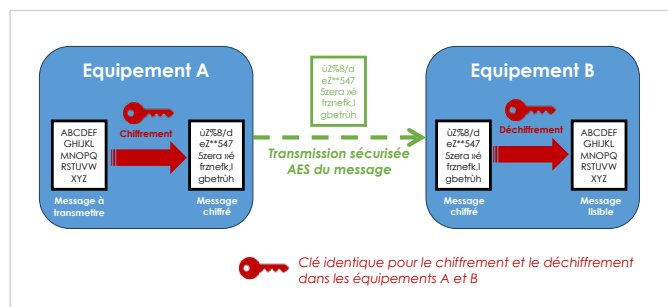
Principe de la communication chiffrée AES
