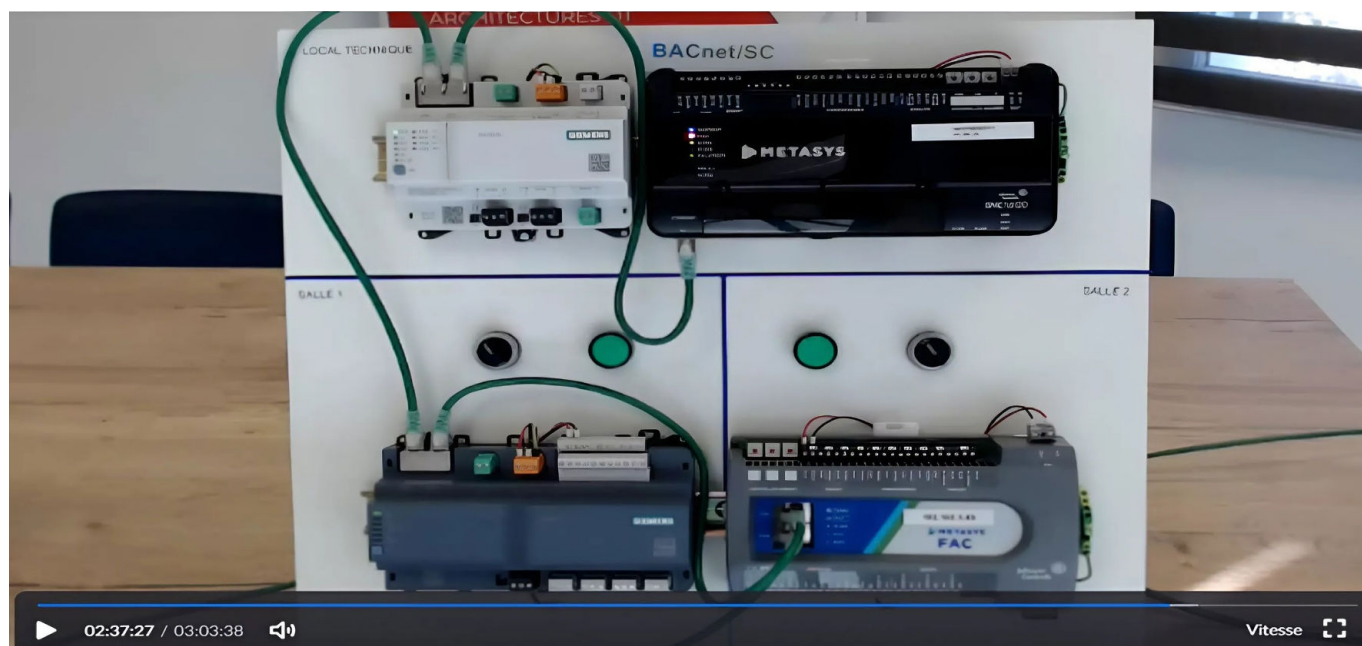
Plateforme physique AGILICOM de tests de mise en œuvre BACnet SC pour les projets multivendors
